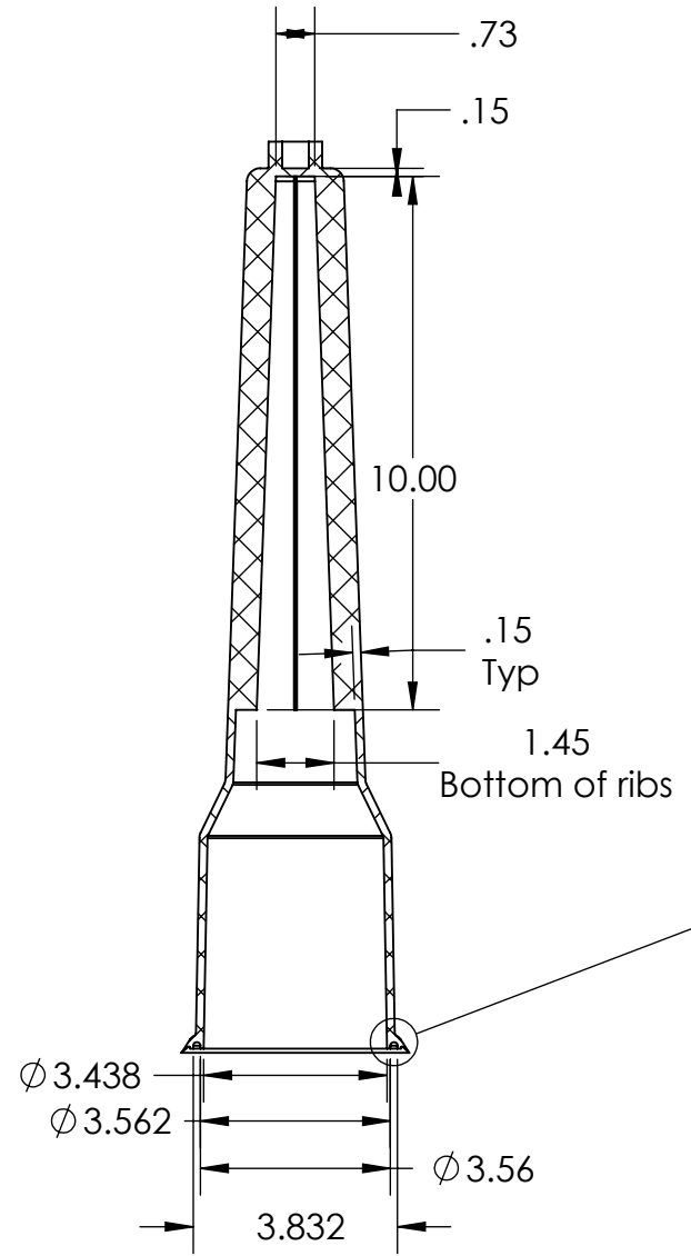
SECTION A-A SCALE 1 : 4
